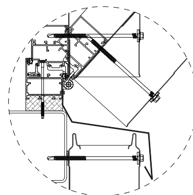
szczegół C
