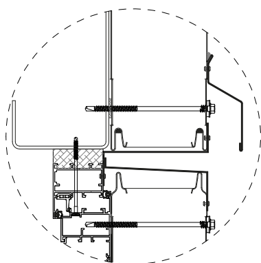
szczegół A
