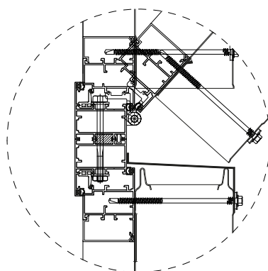
szczegół B
